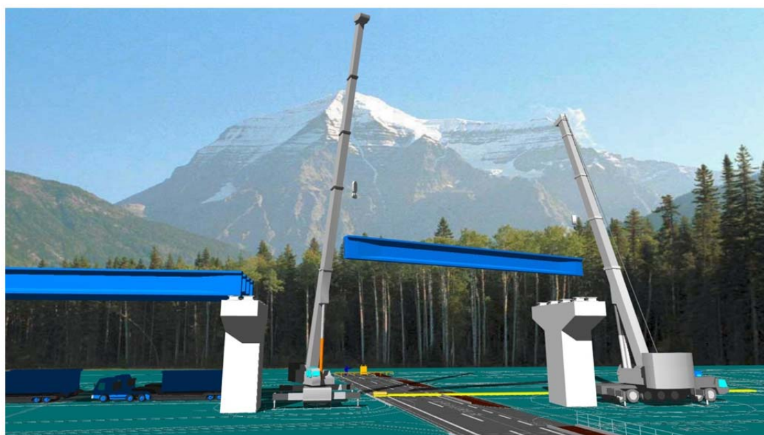
図. 橋梁架設シミュレーションの事例
